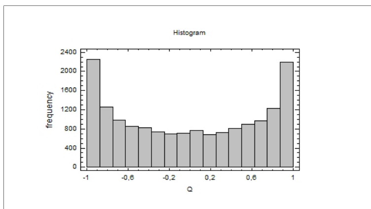
Obrázek 9: Histogram koeficientu asociace Q(A, B) .
