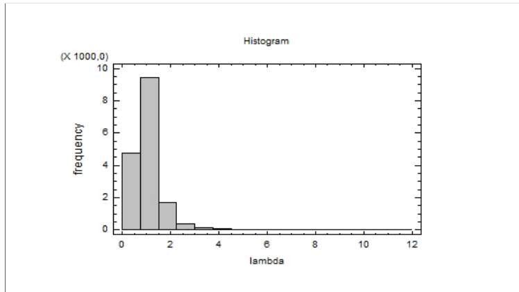
Obrázek 2: Histogram koeficientu koherence \lambda(A, B) .
