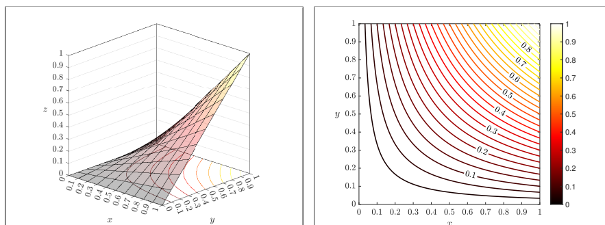
Obrázek 11: Graf a vrstevnice plochy z = xy .
