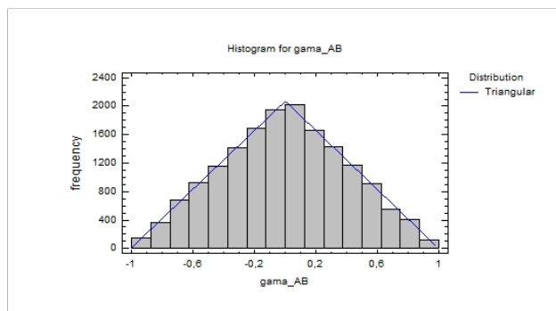
Obrázek 7: Regresní koeficient \gamma_B(A) .
