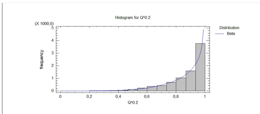
Obrázek 10: Hustota rozdělení veličiny Q^* = |Q(A, B)|^{0,2} .
