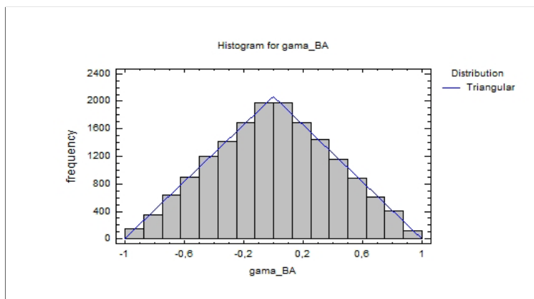
Obrázek 8: Regresní koeficient \gamma_A(B) .
