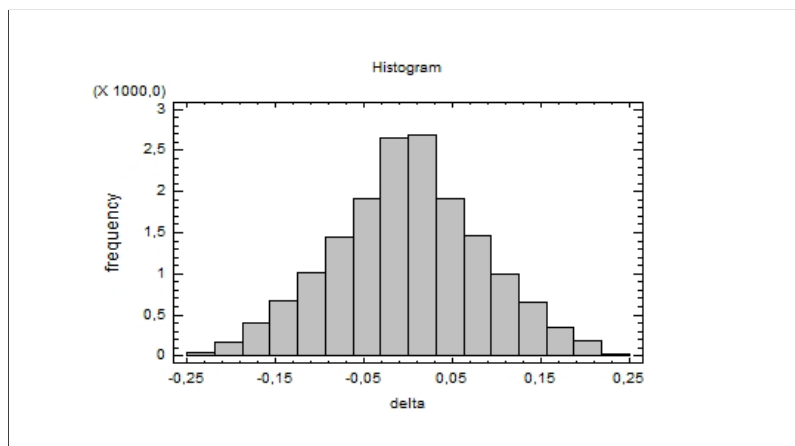
Obrázek 4: Histogram koeficientu kompatibility \delta(A, B) .
