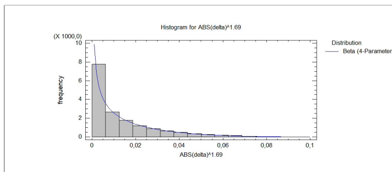
Obrázek 5: Hustota rozdělení veličiny \delta^*(A, B) = |\delta(A, B)|^{1,69} .
