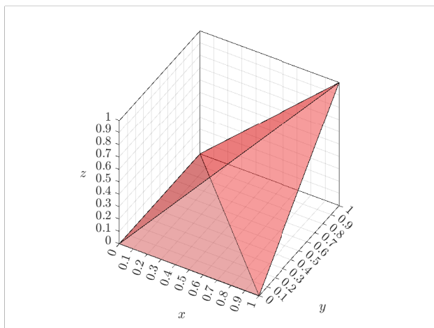
Obrázek 1: Množina M přípustných bodů pro náš model.
