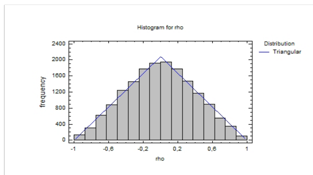
Obrázek 6: Koeficient korelace \rho(A, B) .
