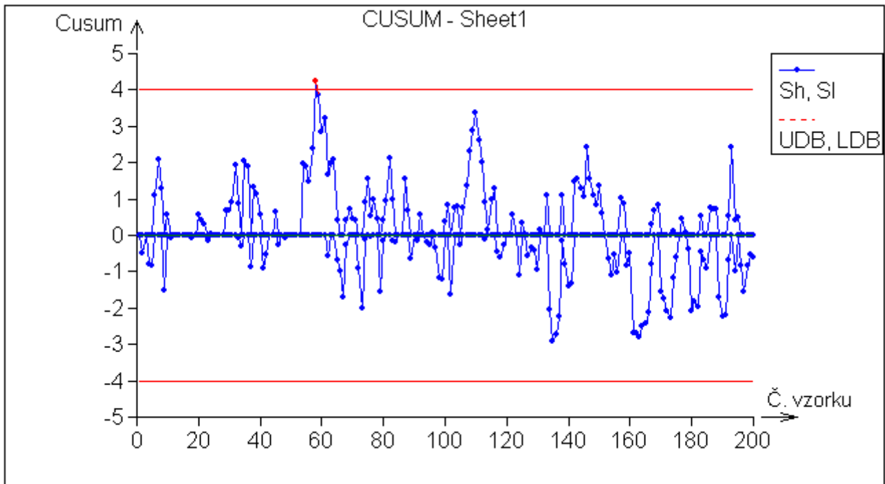
Obrázek 4: Diagram CUSUM
