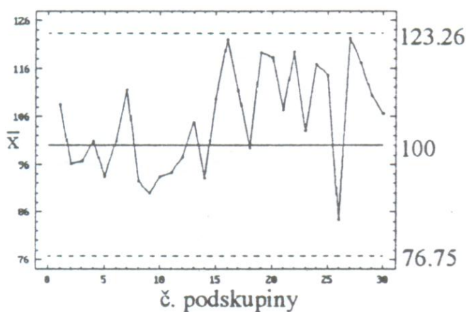
a) Klasický Shewhartův diagram
