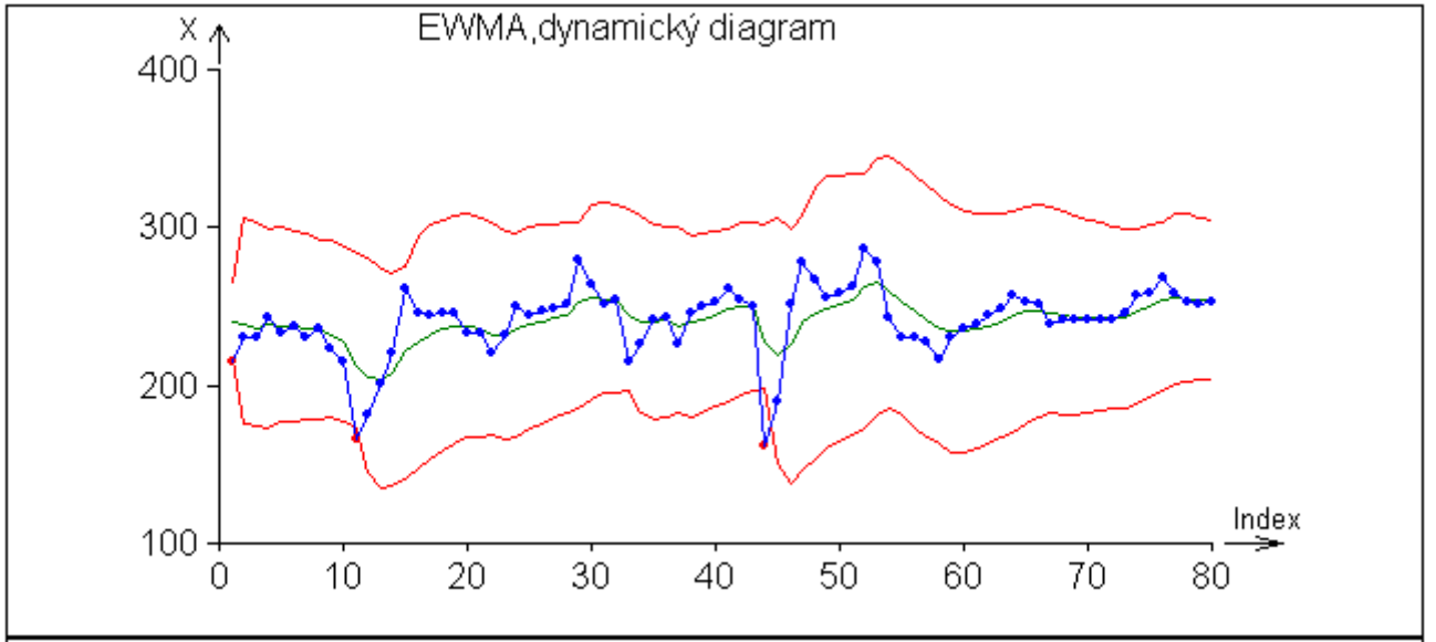
Obrázek 7: Dynamický diagram EWMA
