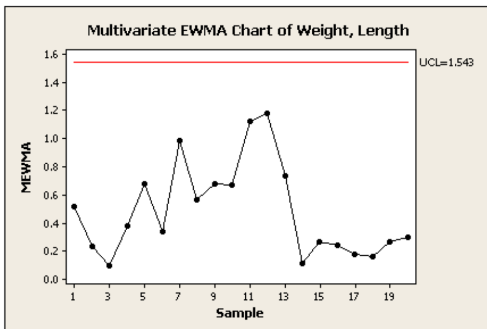
Obrázek 9: Diagram MEWMA
