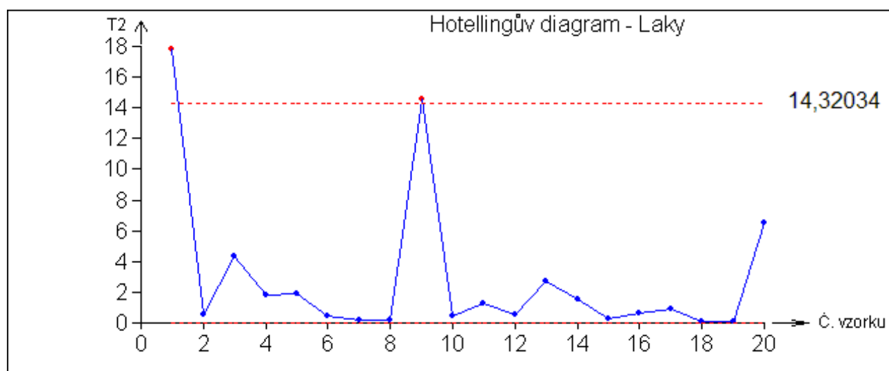
Obrázek 10: Hotellingův diagram
