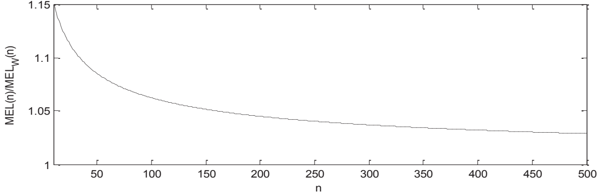
Obrázek 4: Poměr střední délky Waldova-Clopperova IO a Waldova IO v závislosti na rozsahu výběru n
