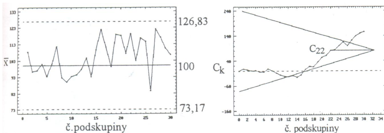
a) Klasický Shewhartův diagram
