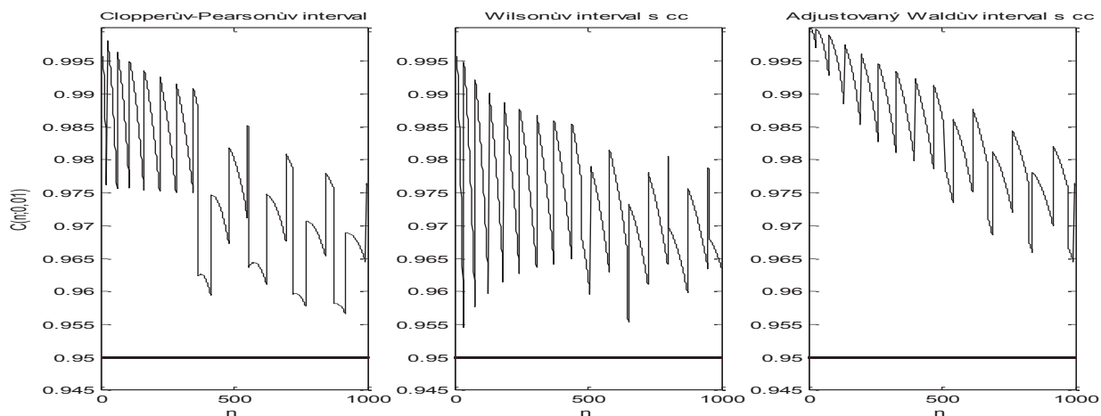
Obrázek 14: Srovnání pokrytí analyzovaných konzervativních intervalů pro \pi = 0,01 , 1 - \alpha = 0,95 a 10 \leq n \leq 1000
