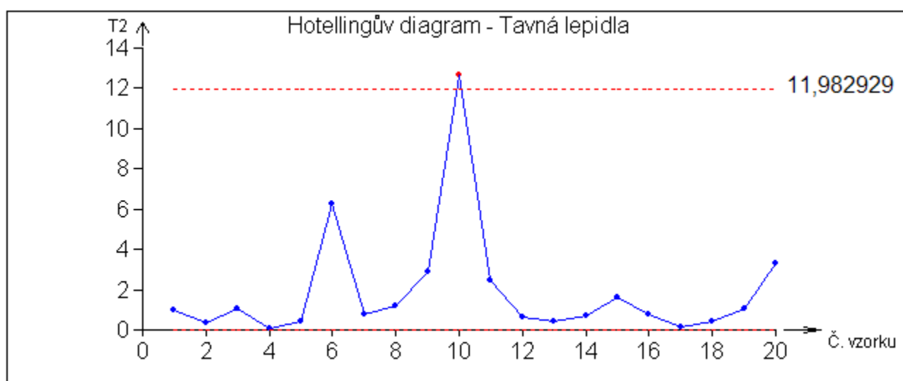
Obrázek 14: Hotellingův diagram
