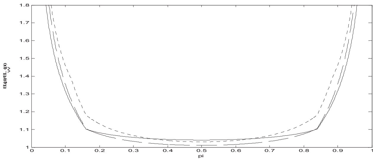
Obrázek 15: Srovnání poměrů délky analyzovaných konzervativních odhadů k délce Waldova intervalu pro n = 20 , 1 - \alpha = 0,95 (Clopper-Pearsonův interval – plná, Wilsonův interval s cc – čerchovaná, adjustovaný Waldův interval – tečkovaná)
