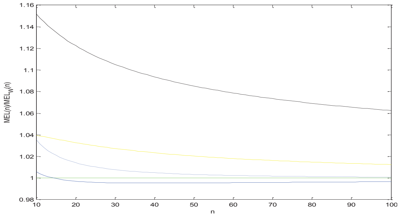
Obrázek 12: Srovnání poměrů střední délky analyzovaných libe- rálních odhadů ke střední délce Waldova intervalu v závislosti na n pro 1 - \alpha = 0,95 (Waldův-Clopperův odhad s cc – černá, arcsi- nový odhad – modrá plná, arcsinový odhad II – modrá čerchovaná, Wilsonův odhad – zelená, adjustovaný Waldův odhad – žlutá).
