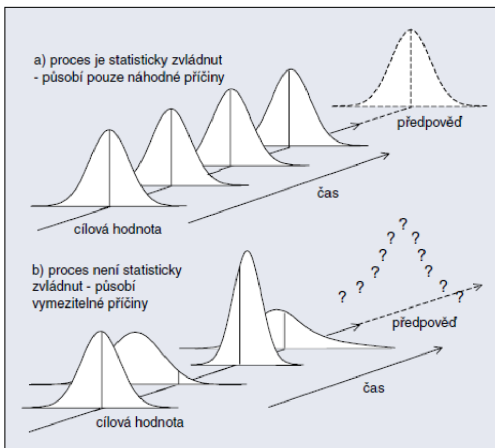
Obrázek 1: Náhodné a vymezitelné příčiny variability
