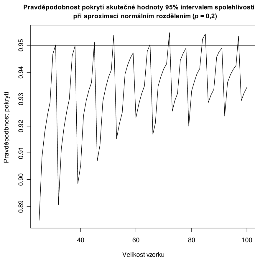
Graf 2.9: Pravděpodobnost pokrytí skutečné hodnoty parametru 95% intervalem spolehlivosti při aproximaci normálním rozdělením pro parametr p = 0,2 při různých hodnotách velikosti vzorku n
