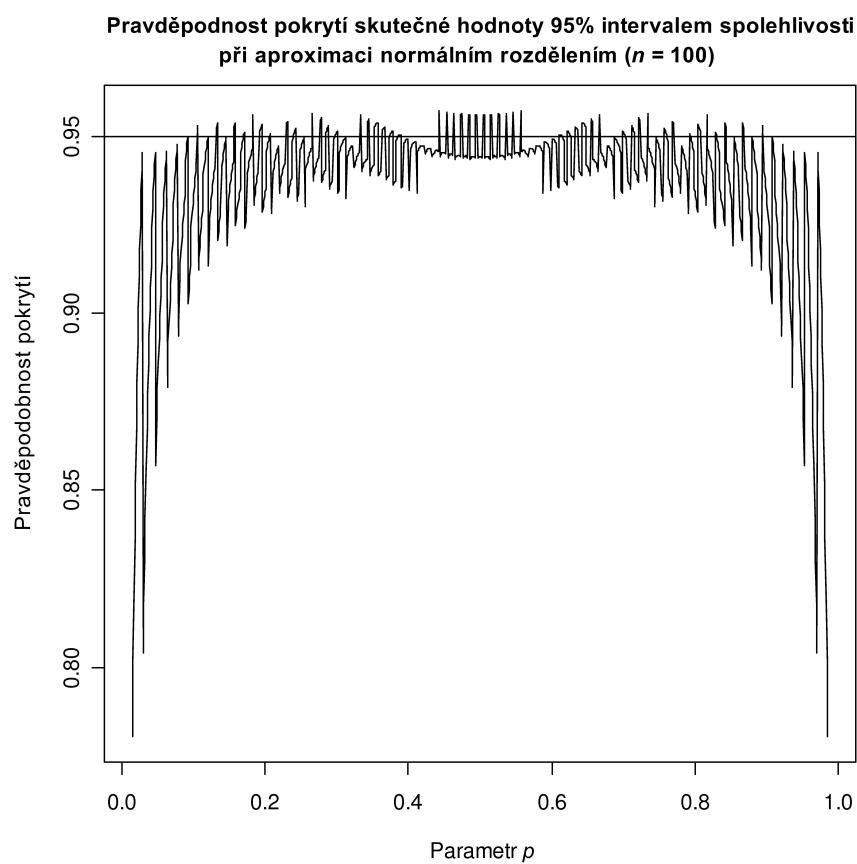
Graf 2.10: Pravděpodobnost pokrytí skutečné hodnoty parametru 95% intervalem spolehlivosti při aproximaci normálním rozdělením pro rozsah výběru (velikost vzorku) n = 100 při různých hodnotách parametru p
