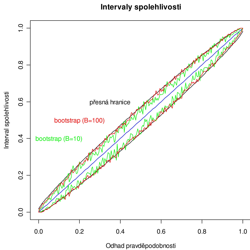
Graf 6.1: Porovnání přesného intervalu spolehlivosti a bootstrapového odhadu
